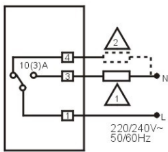
TR-010(T6360A)
