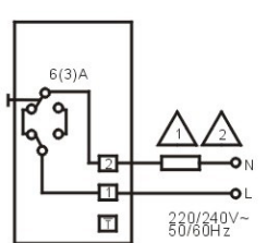
TR-100(T4360D)
